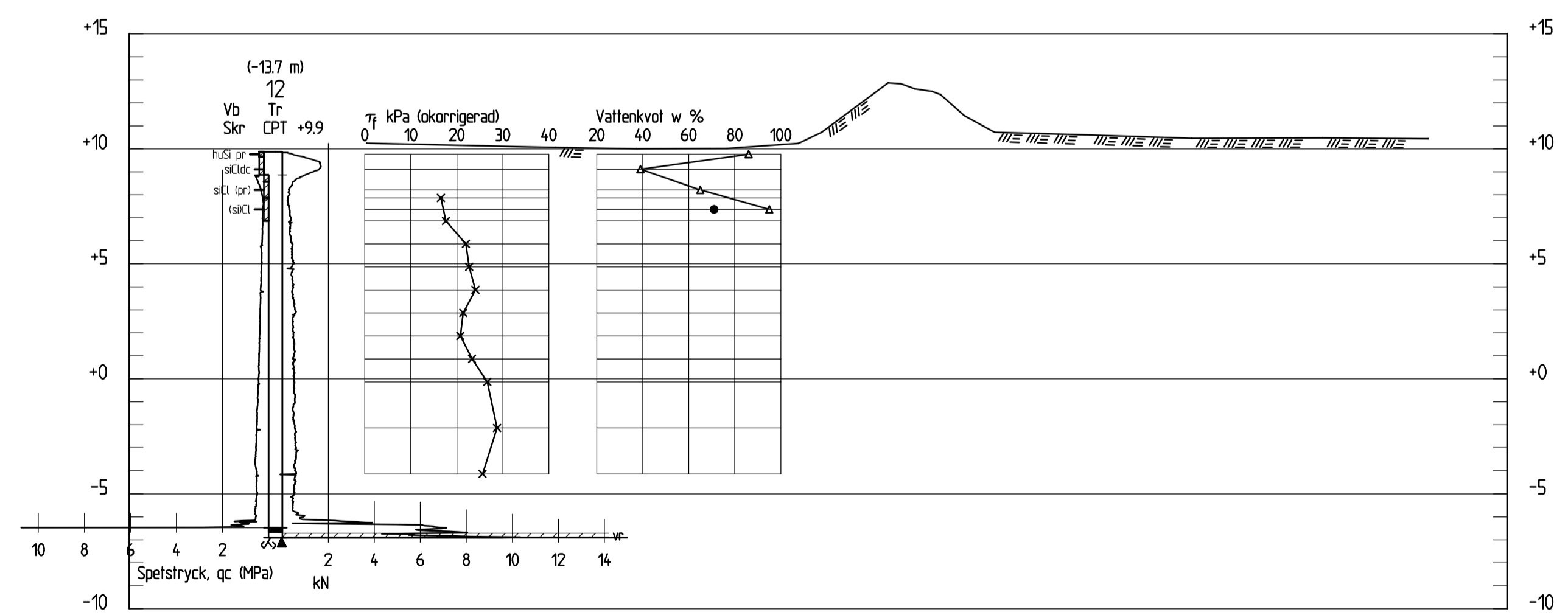
SEKTION C-C 1: 200
